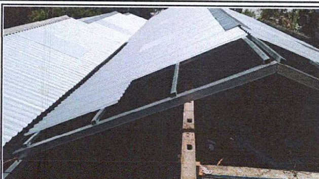
Foto 2: TRABAJO EN PROCESO CUBIERTA DE LAMINAS Y ESTRUCTURA DE TECHO, AULA DE SEGUNDO
